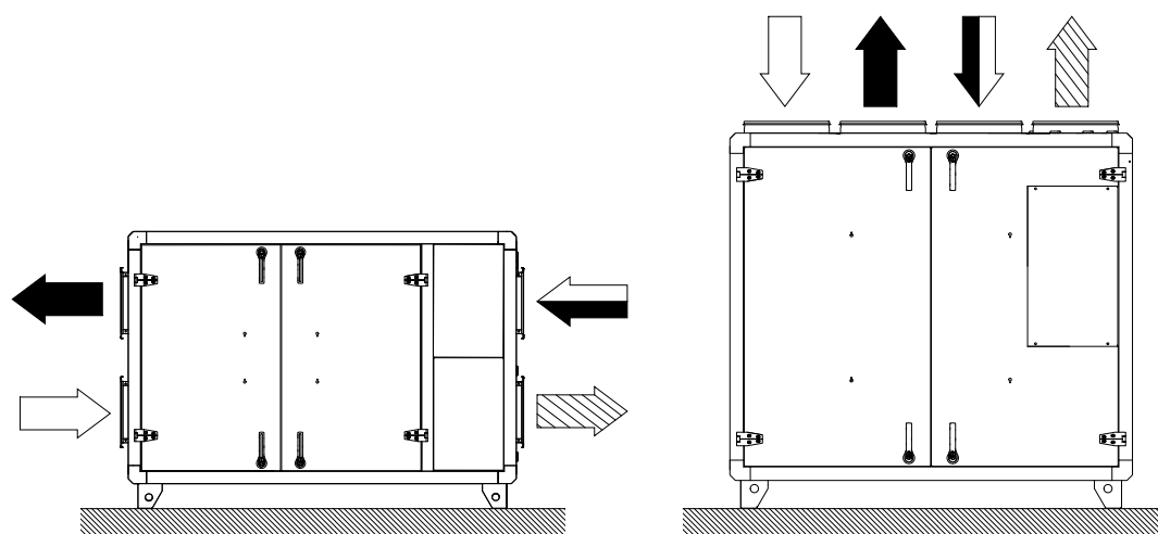
Рис. 8 Монтажное положение (агрегат с левым подключением)
