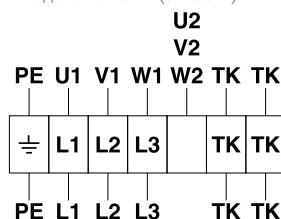
Подключение Y (3~400 В)
