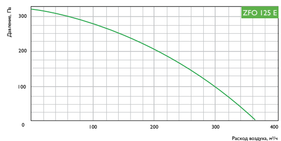
Условия испытаний 150 м³/ч, 210 Па
