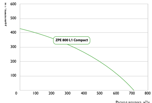
Для ZPE 800 LI Compact
