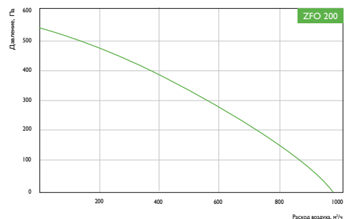
Условия испытаний 600 м³/ч, 240 Па
