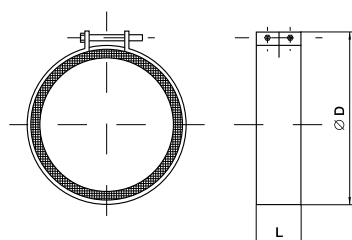
Габаритные размеры
