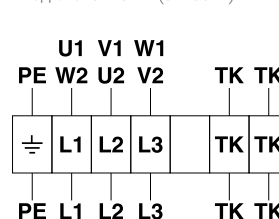
Подключение Δ (3~230 В)
