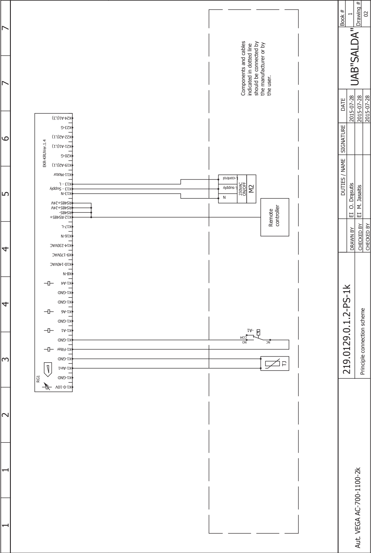
Схема электрического подключения VEGA 700E/1100E AC
