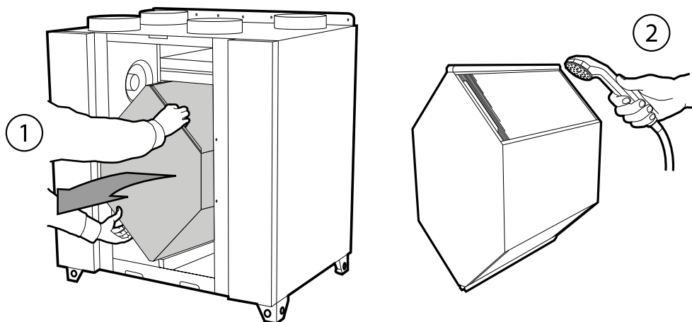
Рис. 8 Снятие и чистка теплообменника
